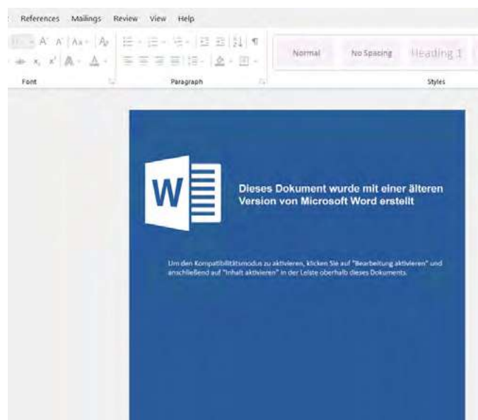
Figure 9. Trojan.VBS.Vshell.A
