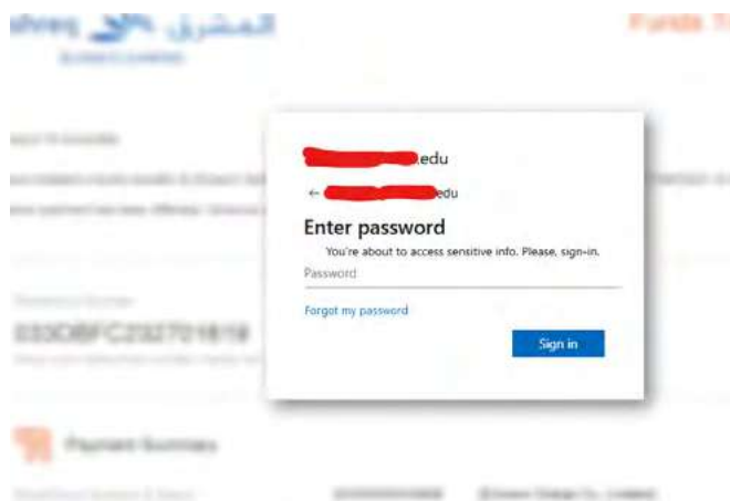
Figure 8. Trojan.HTML.Hidden.1
